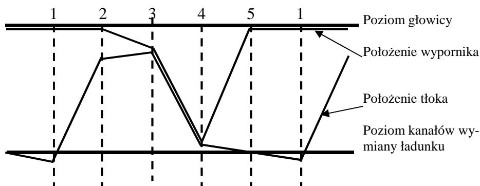
Rys. 2. Przemieszczenia tłoka i wypornika w idealnym silniku z regeneracją ciepła
